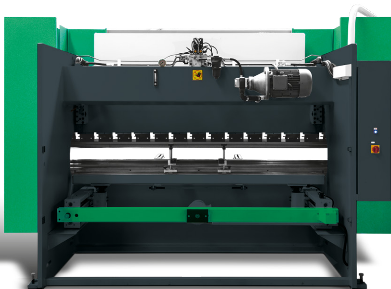
HM CNC HPB 170 - Back
